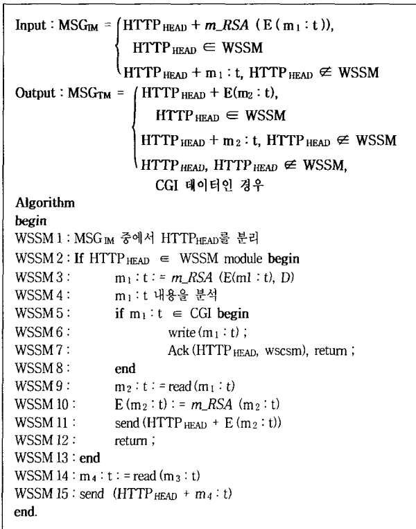
(알고리즘 1) WSSM 보안 모듈의 동작
