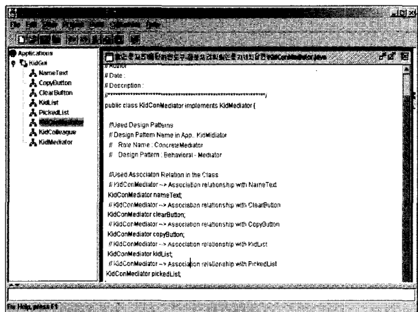
(그림 16) 위저드를 통해 얻어진 소스코드
