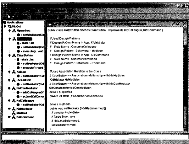
(그림 23) 두 패턴의 역할이 포함되어 자동 생성된 CopyButton 클래스
