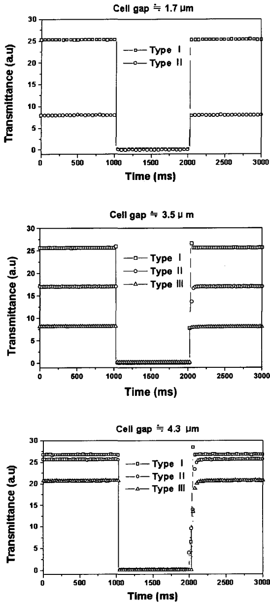
그림 2. 러빙 처리된 PI 표면에 네마틱 액정 및 셀 갭 d에 따른 TN 셀의 응답 특성. Fig. 2. Response characteristics of the TN cell with different NLCs and cell gap d on the rubbed PI surface.
