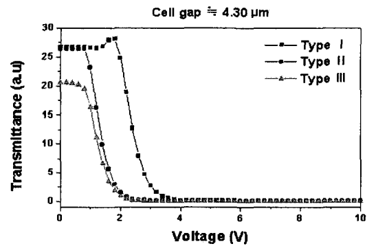
그림 1. 러빙 처리된 PI 표면에서 네마틱 액정 및 셀갭 d에 따른 TN 셀의 전압-투과율 (V-T) 특성.
