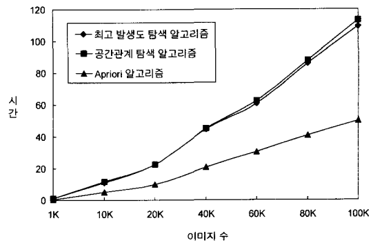
그림 2. 알고리즘별 평균 실행시간
