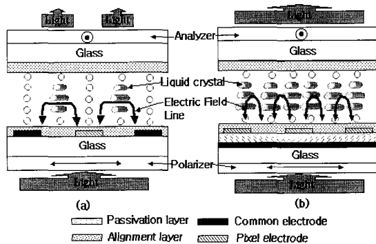
그림 1. On 상태에서 액정분자들의 구조를 갖는 (a) IPS 셀 구조나 (b) FFS 셀 구조의 단면도. Fig. 1. Cross-sectional view of (a) the IPS and (b) the FFS cell structures with configuration of the LC molecules in on state.
