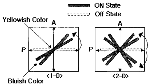
그림 3. 1-D와 2-D를 갖는 FFS 모드에서 Off와 On 상태에서 액정 방향자의 형태.
