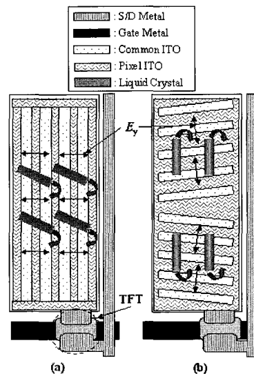
그림 2. (a) 1-D나 (b) 2-D에 대해 TFT를 갖는 FFS 소자의 단위 화소 구조. Fig. 2. One pixel structure of the FFS device with TFT for (a) 1-D and (b) 2-D.
