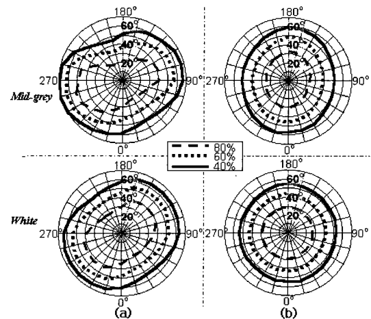
그림 4. 중간 계조와 밝은 계조에서 (a) 1-D와 (b) 2-D를 갖는 FFS 모드의 등 휘도 곡선.
