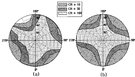
그림 5. (a) 1-D와 (b) 2-D를 갖는 FFS 모드의 등-콘트라스트 곡선.
