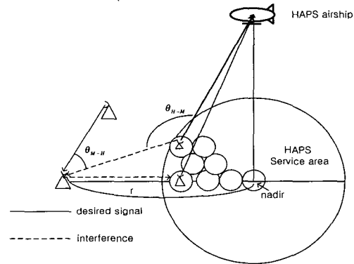
그림 4. HAPS 지구국이 무선 중계국에 미치는 간섭
