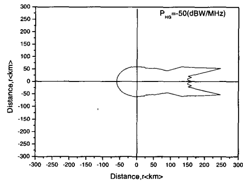
그림 11. 무선 중계국과 HAPS nadir간의 조정 거리
