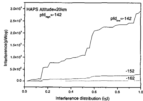
그림 8. pf_{low} 에 따른 간섭 분포
