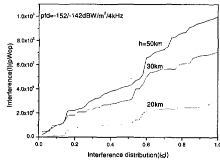
그림 6. HAPS 고도에 따른 간섭 분포
