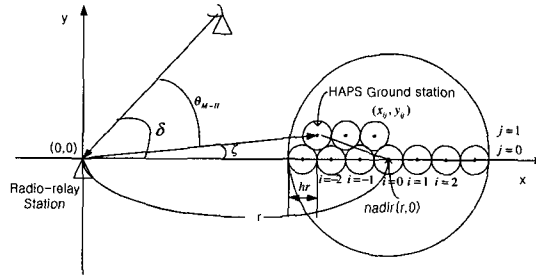
그림 5. \theta_{M-H} 와 \theta_{H-M} 을 구하기 위한 모델
