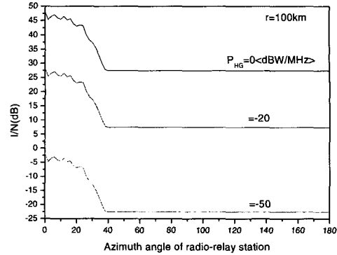
그림 9. 전송 전력 밀도 P_{HG} 에 따른 I/N
