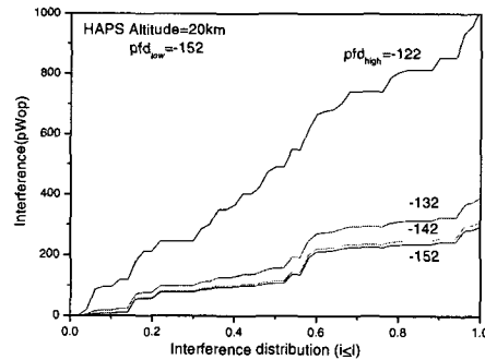
그림 7. pf_{high} 에 따른 간섭 분포
