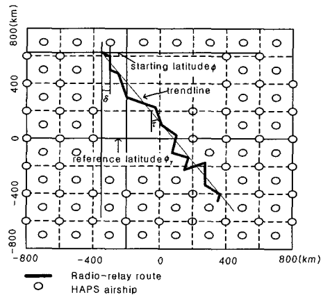
그림 1. 무선중계국과 HAPS airship의 분포
