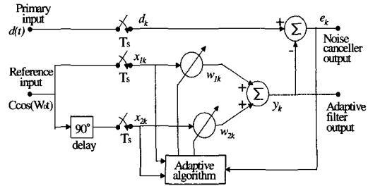
그림 1. 적응 노치 필터의 구조
