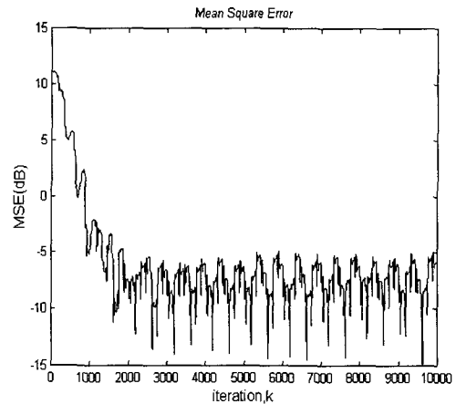
그림 9. VSS LMS 알고리즘의 MSE 곡선
