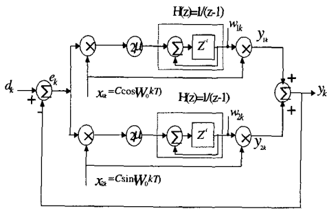
그림 2. LMS 적응 노치 필터의 흐름도
