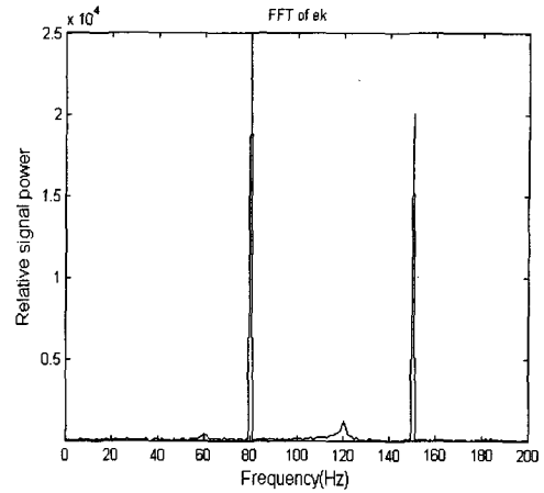
그림 10. 상관 추정 LMS 알고리즘의 출력신호 주파수
