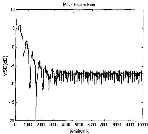
그림 7. LMS 알고리즘의 MSE 곡선
