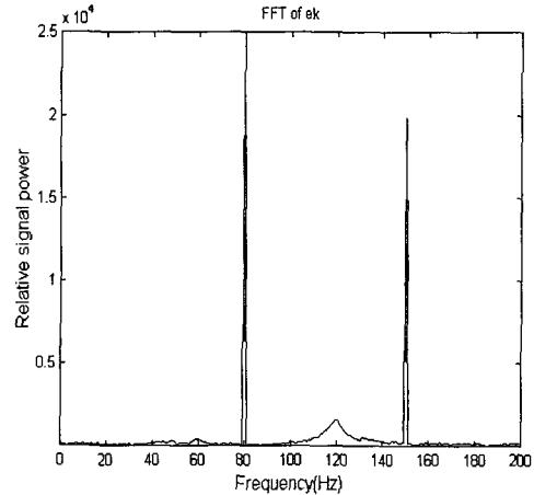
그림 8. VSS LMS 알고리즘에서 출력신호의 주파수 스펙트럼
