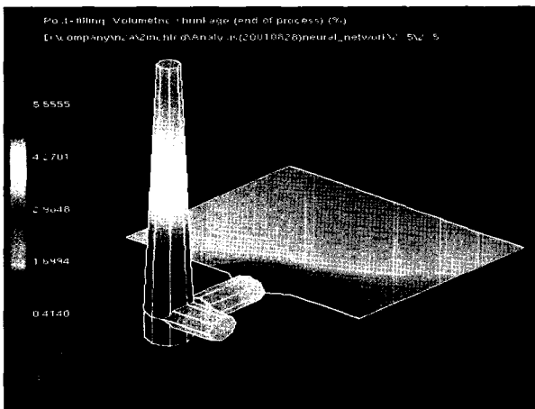
<그림 3> 기존의 조건에 의한 체적 수축률
