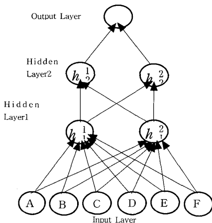
<그림5> 역전파 신경망 설계
