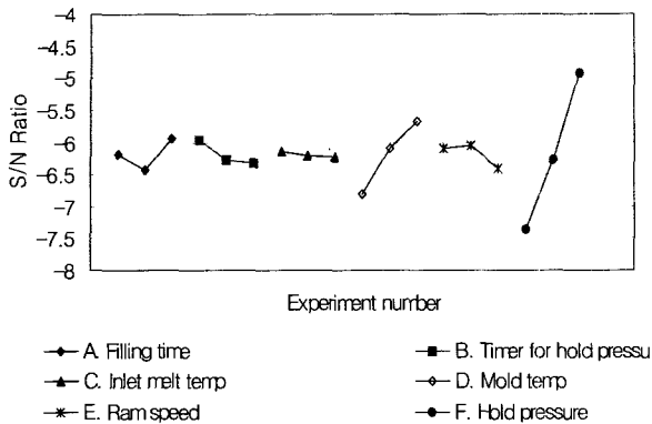
<그림 2> 인자의 수준별 평균값
