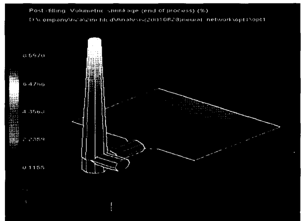
<그림6> 신경망이론에 의한 체적 수축률
