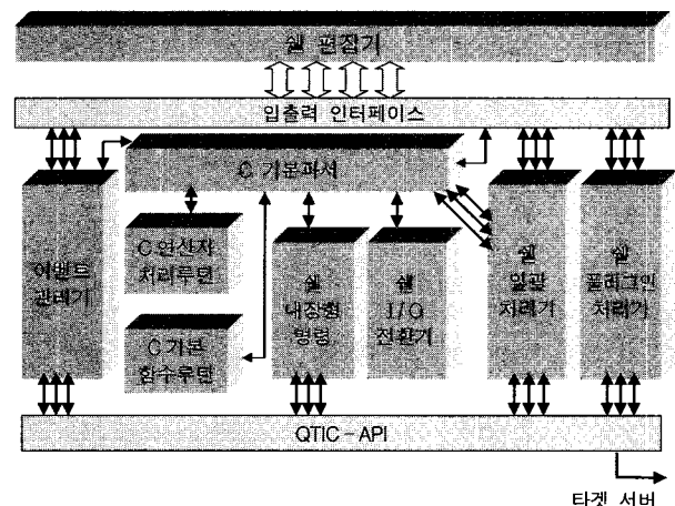
(그림 4) 대화형셸 구조도
