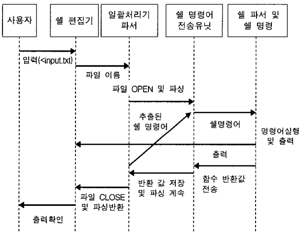
(그림 10) 일괄처리 기능의 흐름도
