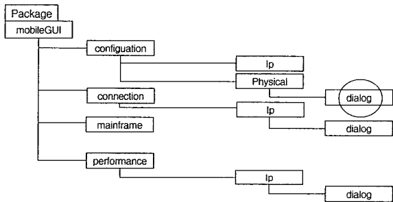
(그림 8) 망관리 사용자 인터페이스의 패키지 상관도
