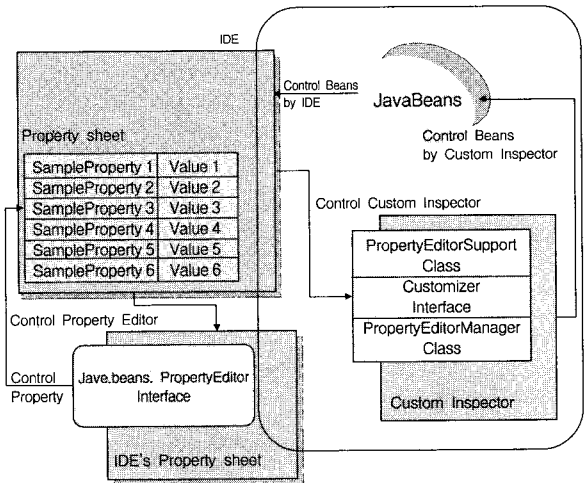
(그림 7) 커스텀 인스펙터에 의한 빈의 제어
