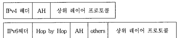
(그림 5) IPv4와 IPv6에서의 AH 구조
