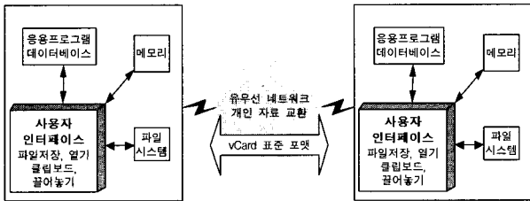
(그림 1) vCard 표준 포맷을 이용한 개인 정보 교환
