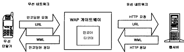
(그림 2) 무선 인터넷 구성
