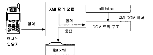
(그림 11) 디렉토리 정보의 전달
