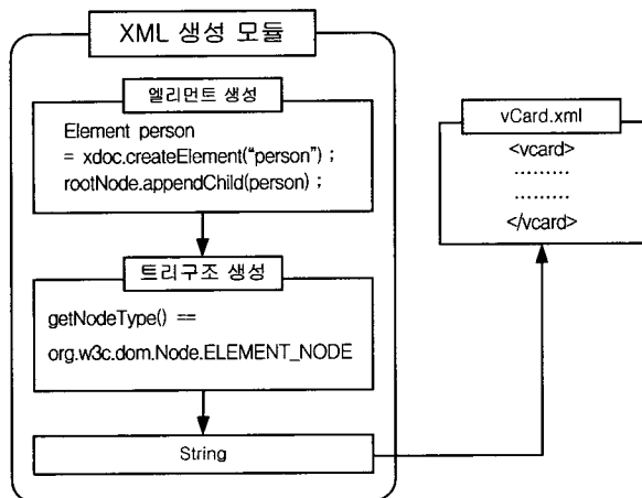
(그림 5) XML 문서의 생성
