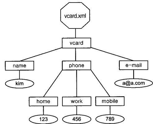
(그림 6) DOM 트리 구조
