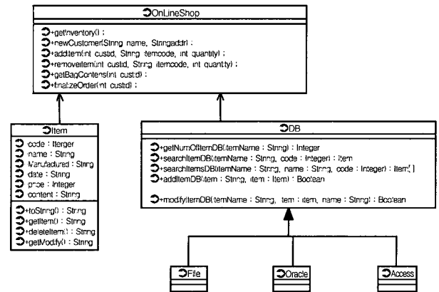
(그림 4) 사례연구 Class Diagram
