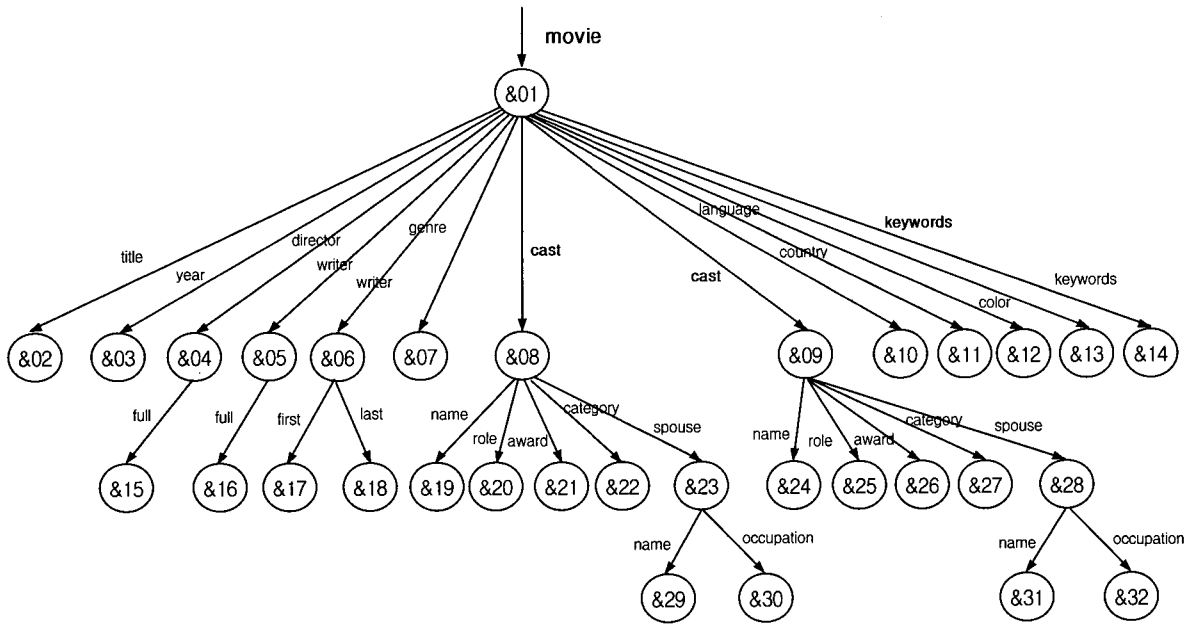
(그림 4.2) XML 문서에 대한 데이터 그래프
