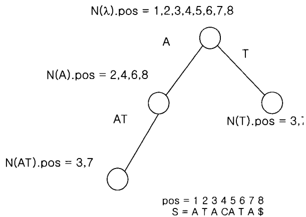
(그림 2) 문자열 "ATACATA"에 대한 Vilo 트리
