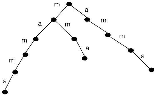
(그림 1) 문자열 "mamma"에 대한 접미사 트리
