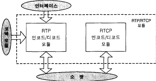
(그림 5) H.323 시스템의 RTP/RTCP 모듈 구성도
