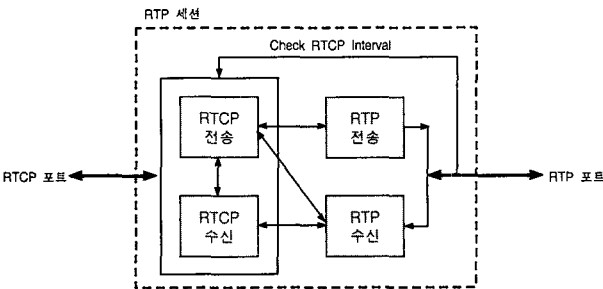
(그림 7) RTP 세션 구성도
