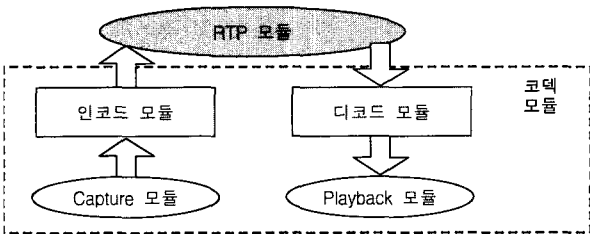
(그림 6) H.323 시스템의 코덱 모듈 구성도
