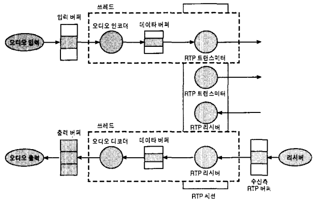
(그림 8) RTP 세션과 오디오 코덱과의 관계 구성도
