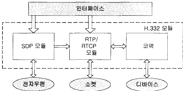
(그림 3) H.332 시스템의 전체 구성도
