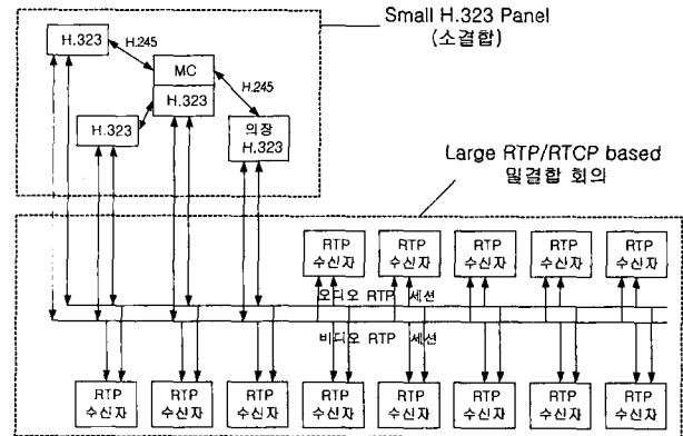
(그림 1) H.332 시스템 구성도
