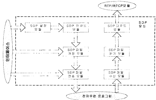
(그림 4) H.332 시스템의 SDP 모듈 구성도
