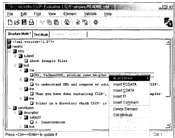
(그림 1) 트리 기반 XML 문서 편집기
