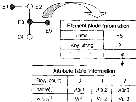
(그림 14) XML AST를 구성하기 위한 노드의 자료구조
