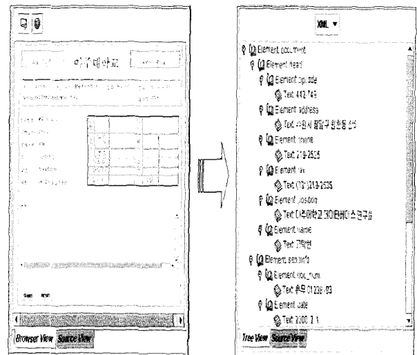
(그림 16) 브라우저에서 입력 form을 통한 XML 문서 생성
