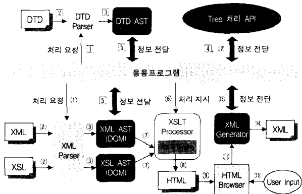
(그림 6) XML 문서 처리 전체 흐름도
