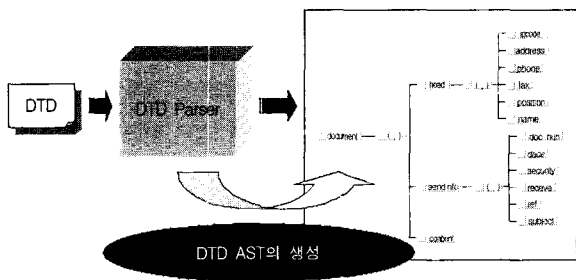
(그림 9) DTD AST의 생성
