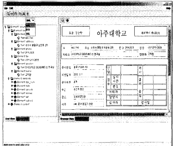
(그림 7) Form 양식을 지원하는 XML 문서 편집기 화면구성
