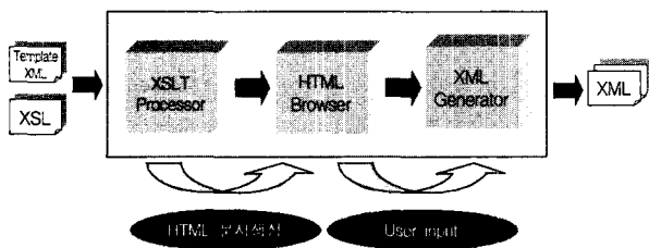
(그림 5) Form-based를 지원하기 위한 시스템 주요 구성도
