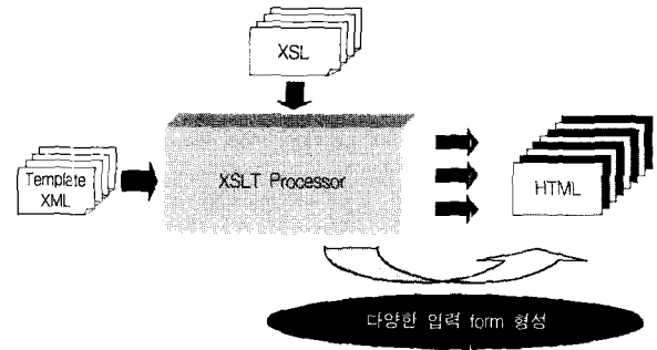
(그림 15) XSLT Processor를 통한 다양한 입력 form 생성
