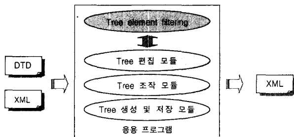
(그림 4) 트리 기반 XML 문서 작성을 위한 구성 요소
