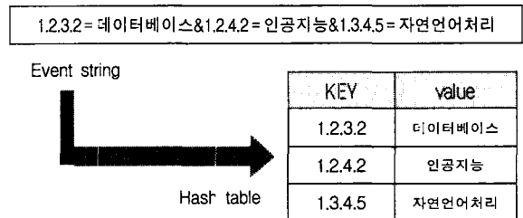
(그림 18) event 스트링에서부터 생성된 해쉬 테이블
