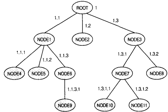
(그림 17) 고유한 경로에 근거한 XML 엘리먼트의 키 값 부여
