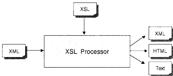
(그림 2) XSLT 문서 처리 흐름
