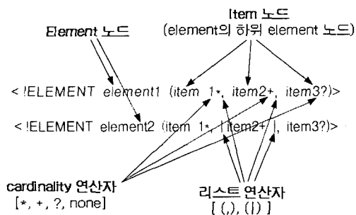
(그림 10) DTD element의 정의
