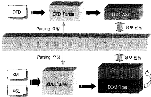
(그림 13) DTD 및 XML 파서 구성도
