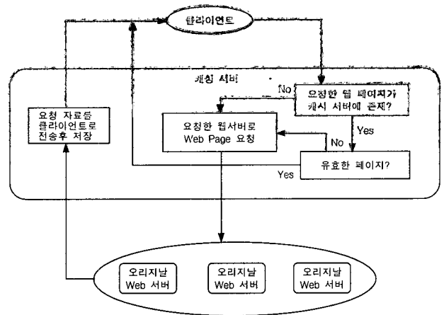
(그림 1) 캐시서버의 흐름도
