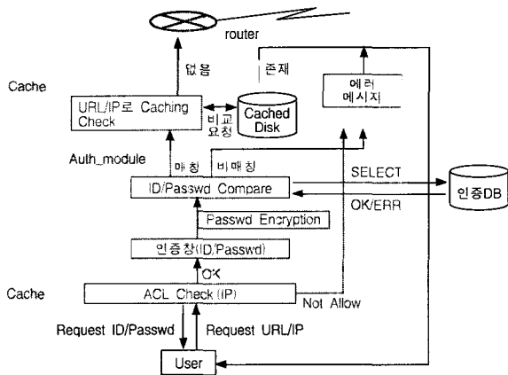
(그림 4) 캐시서버와 인증모듈간의 작업 흐름도
