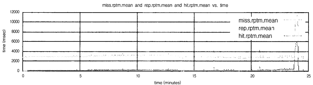
(그림 8) 캐시 응답시간
