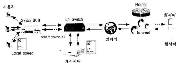
(그림 2) 투명 캐시 구성 및 흐름도
