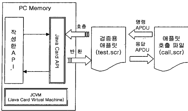
(그림 8) 검증 애플릿 실행 구조
