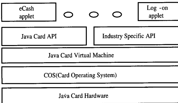
(그림 1) 자바 카드 구조
