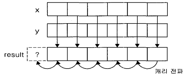
(그림 6) 기본 연산 구조도
