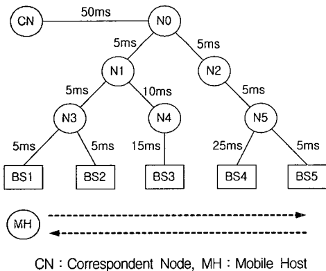
(그림 9) 실험 토폴로지 2
