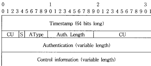
(그림 4) Cellular IP Routing Update Message Payload Format
