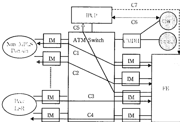
(그림 4) MPLS ATM (LER) 시스템의 논리적인 구성도
