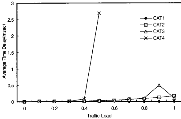
(그림 11) 응용 범주별 지연 시간
