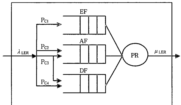
(그림 10) 포워딩 엔진 시뮬레이션 모델
