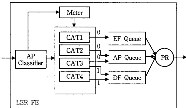
(그림 9) 응용 기반 포워딩 엔진 모델
