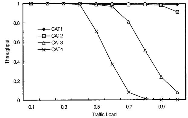
(그림 13) 응용 범주별 처리율
