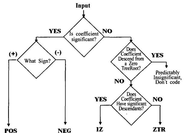
(그림 10) Dominant 단계에서 심벌이 부호화 되는 과정의 흐름도
