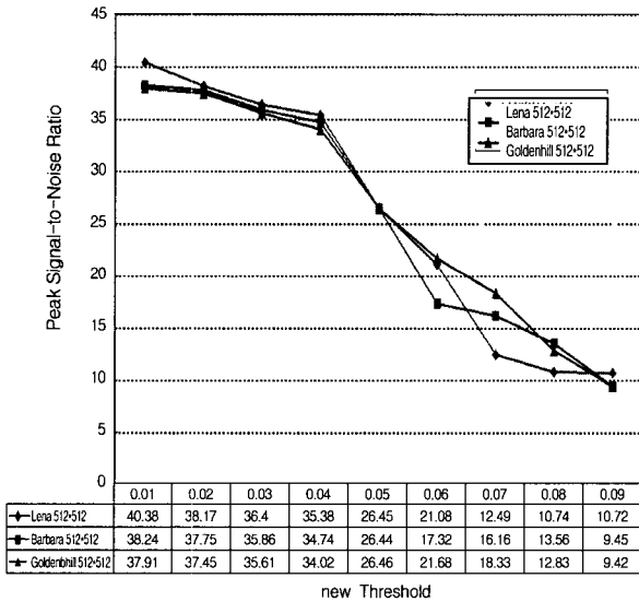
(그림 18) 원 영상과 복원 영상의 PSNR 비교
