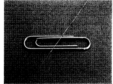
그림 2 병간에서 압출된직경 200 \mu m 세선, 초기 소재의 직경은 1mm
