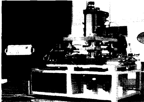
그림 3 미세 복합 성형 프레스(한국생산기술연구원)
