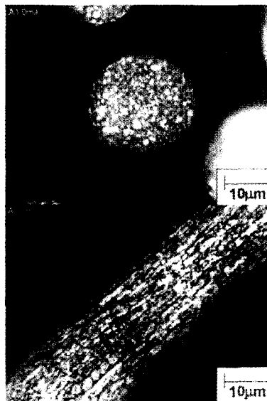
그림 7 Gold bonding wire 직경 24 \mu m, 결정립 크기 0.3 \mu m
