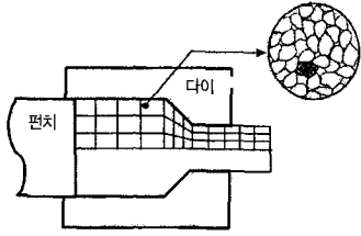
그림 8(a) 다결정 해석
