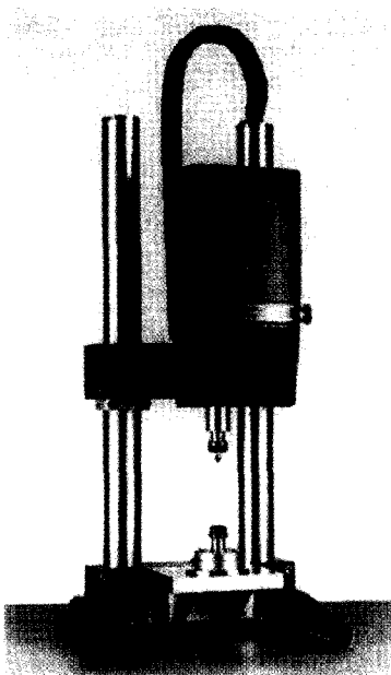
그림 6 미세인장시험기(instron 8848)
