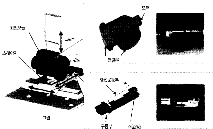
그림 5 정밀위치 결정기구의 구성
