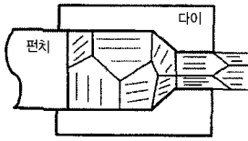
그림 8(b) 메조 스코픽 해석
