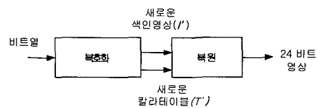
그림 4. 색인 재배치 복호화
