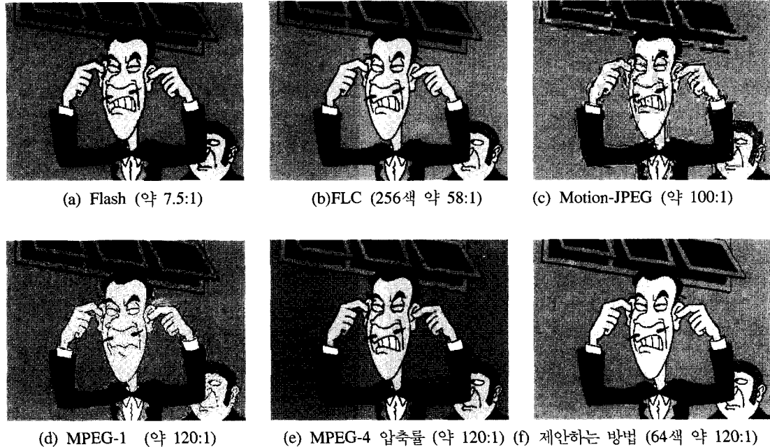
그림 8. 제안하는 방법과 다양한 방법의 비교
