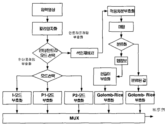
(a) 부호화 알고리즘
