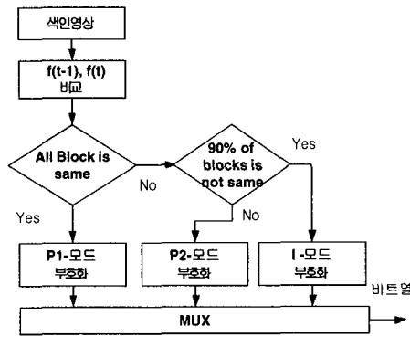
그림 7. 인터 프레임 모드
