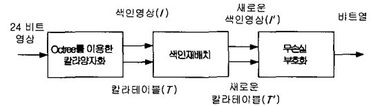
그림 3. 색인 재배치 부호화
