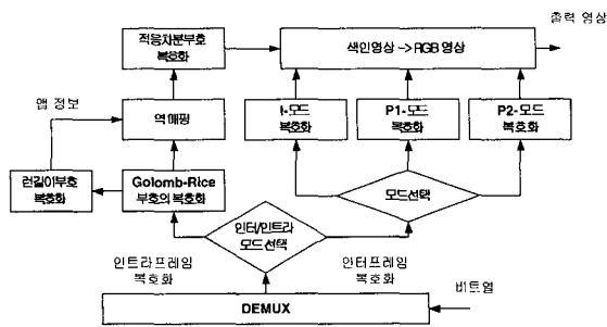
(b) 복호화 알고리즘
