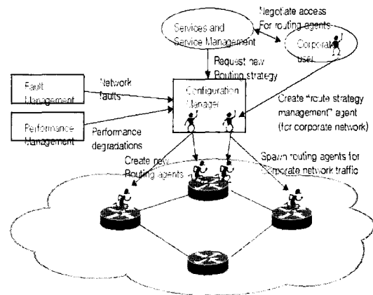
그림 2. MIAMI 플랫폼의 구조
