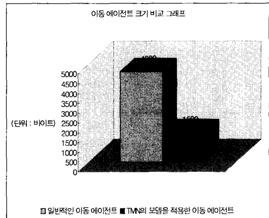
그림 12. 이동 에이전트 코드 크기 비교 그래프
