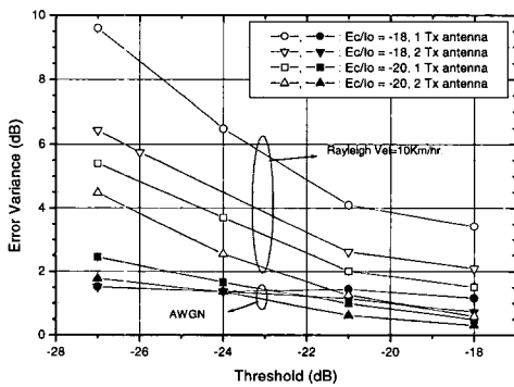
그림 6. 제 1차 드웰 임계치 \delta_1 에 따른 제한된 E_c/I_0 예측기의 예측오차의 분산 컴퓨터 모의실험 결과 ( \delta_v 은 -27 dB). (10 \log_{10}(E_c/I_{cr}) = 10 \log_{10}(E_c/I_{cr}) + 10 \log_{10}(I_{cr}/I_{cr}) )
