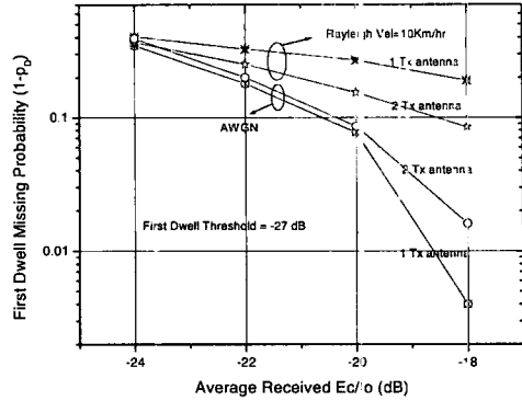
그림 8. 수신 E_c/I_o 에 따른 제 1차 드웰 실패확률 컴퓨터 모의실험 결과
