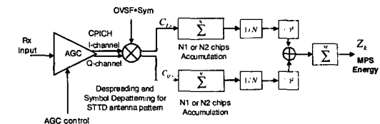
그림 2. MPS 수신모델 (수신 다이버시티 사용시에는 수신 AGC 앞단부터 수신 안테나 2에 대하여 같은 구조가 추가되고 각각 넌코히어런트 결합이 된다)
