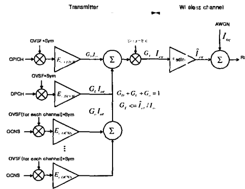
그림 1. 전송 및 채널 모델 (전송 다이버시티 사용시에는 스크램블 앞단에 전송 안테나 2에 대하여 같은 구조가 추가된다)
