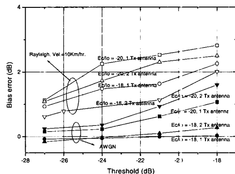
그림 5. 제 1차 드웰 임계치 \delta_1 에 따른 제안된 E_c/I_o 예측기의 바이어스오차 컴퓨터 모의실험 결과 ( \delta_1 은 -27 dB).
