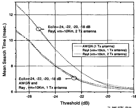
그림 10. 제 1차 드웰 임계치에 따른 평균 탐색시간 컴퓨터 모의실험 결과 (Simulation results for the MPS mean search time vs. \delta_{11} , \delta_{12} is -27 dB).
