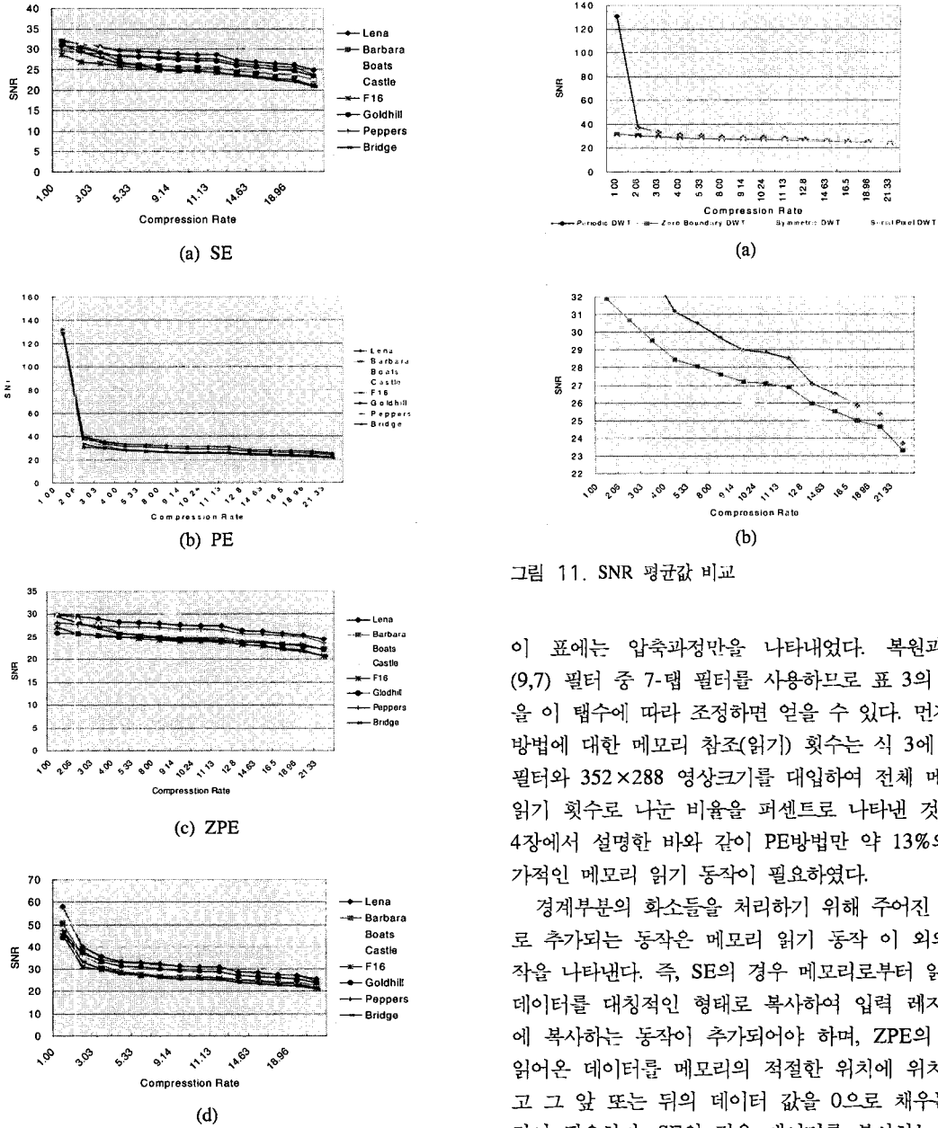
그림 10. 네 방법의 압축률 증가에 따른 SNR 변화
