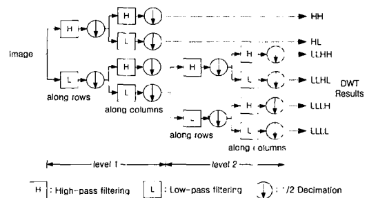
그림 2. 2차원 DWT의 2-레벨 수행절차
