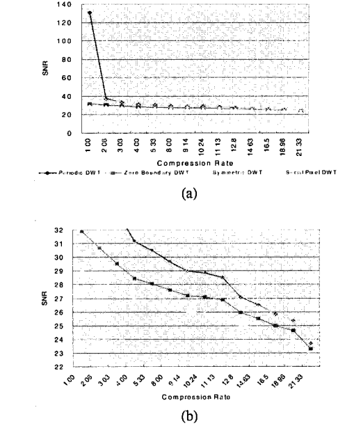
그림 11. SNR 평균값 비교
