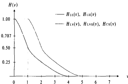
그림 5. LL와 LH 및 LV, LVH와 CH 클래스의 수평 전달함수
