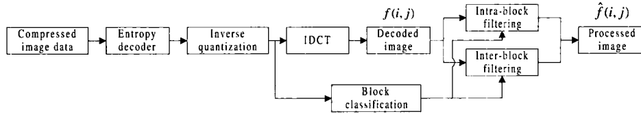
그림 1. 제안한 블록화 현상 제거 방법의 블록도
