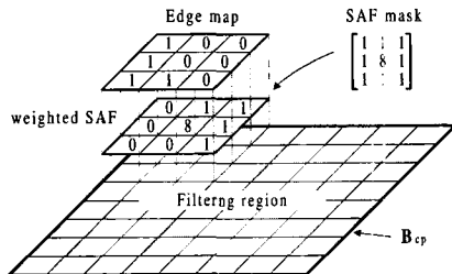
그림 7. SAF를 이용한 블록 내 필터링
