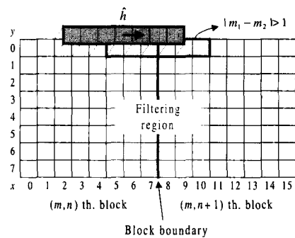
그림 6. 매우 평탄한 블록들간의 \hat{h}_7 을 이용한 블록간 필터링 ( \alpha = 2 ).
