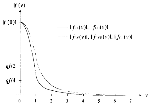
그림 4. qf 가 32와 48로 JPEG 부호화된 LENA 및 BOAT 영상에 대한 LL, LV, LH, LVH, 및 CH 클래스들의 대표적인 1D 최대 수평 주파수 분포
