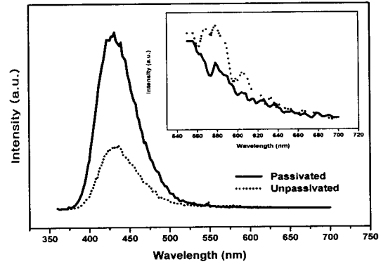
그림 3 600°C에서 어닐링한 실리콘 박막의 수소 passivation 전후의 PL 스펙트럼. (삽입 그림은 500nm 이상의 파장 영역을 확대하여 다시 그린 PL 스펙트럼) Fig. 3 Room temperature PL spectra of Si samples after annealing at 600°C in N 2 for 10 minutes and after an additional annealing at 500°C in forming gas (95 % N 2 + 5 % H 2 ) for 1 hr.
