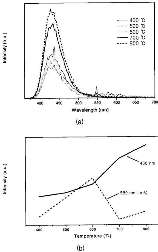
그림 2 어닐링 온도변화에 따른 실리콘 박막의 PL 스펙트럼. Fig. 2 PL spectra from Si nanocrystals annealed at the various annealing temperatures. All samples were annealed in N 2 ambient for 10 minutes.
