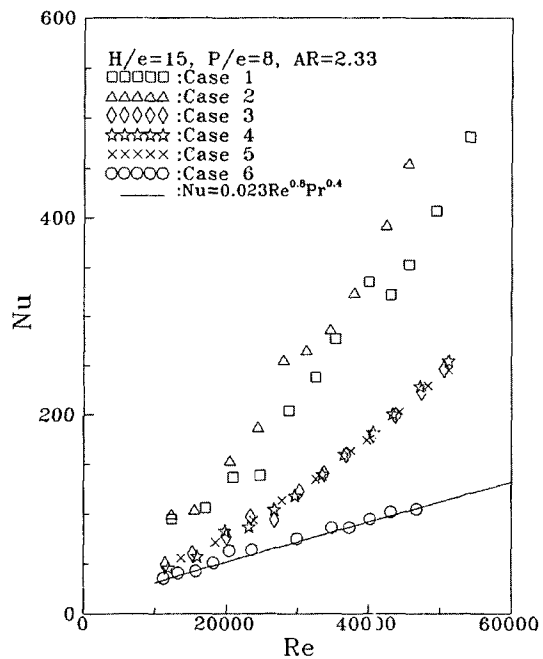
Fig. 4 Nusselt number
