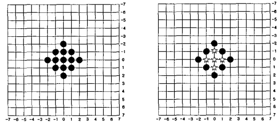
(A) 초기 탐색점 (B) 마지막 단계 (C) 최소 블록 오차를 가진 점의 위치가 상, 하, 좌, 우 방향에 있는 경우 추가 탐색점의 위치 (D) 최소 블록 오차를 가진 점의 위치가 대각선 방향에 있는 경우 추가 탐색점의 위치 (그림 3) 수정된 다이아몬드 탐색 기법(참조 프레임의 움직임 벡터가 (0,0)이 아닐 때 사용)
