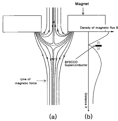
그림 5. 자력선 분포와 자속 밀도 분포. (a) Toroidal 자석의 중심 부분에서 관측되는 자력선 분포. (b) 중심축 방향의 자력선 분포와 초전도체에 작용하는 자기력.
