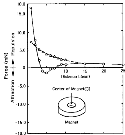
그림 4. 시료와 자석과의 거리에 대한 자기력 변화.
