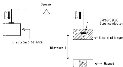
그림 3. 자기력 측정장치.
