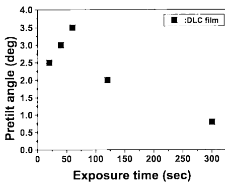
그림 5. DLC 박막 표면에 IB 조사시의 조사시간에 따른 네마틱 액정의 프리틸트각의 발생.
