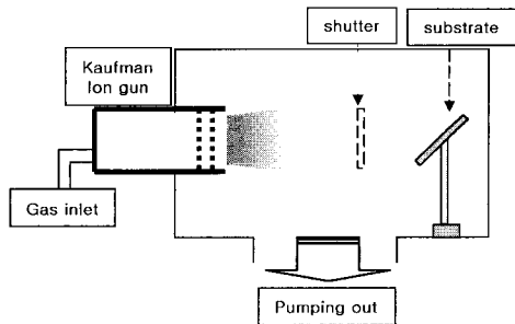
그림 1. IB 조사 시스템. Fig. 1. IB exposure system.
