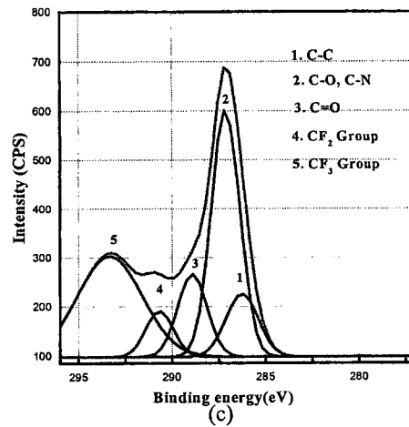
그림 4. (a) 식각전 PI 박막 표면 (b) O 2 /CF 4 =8/2 (c) CF 4 가스로 식각된 PI박막 표면에서의 C 1s 의 XPS narrow scan 스펙트럼.
