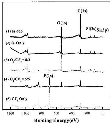
그림 3. PI 박막의 XPS wide scan Spectrum. Fig. 3. XPS wide scan spectra of PI film surface etched under CF 4 /(CF 4 +O 2 ) gas mixing ratio.
