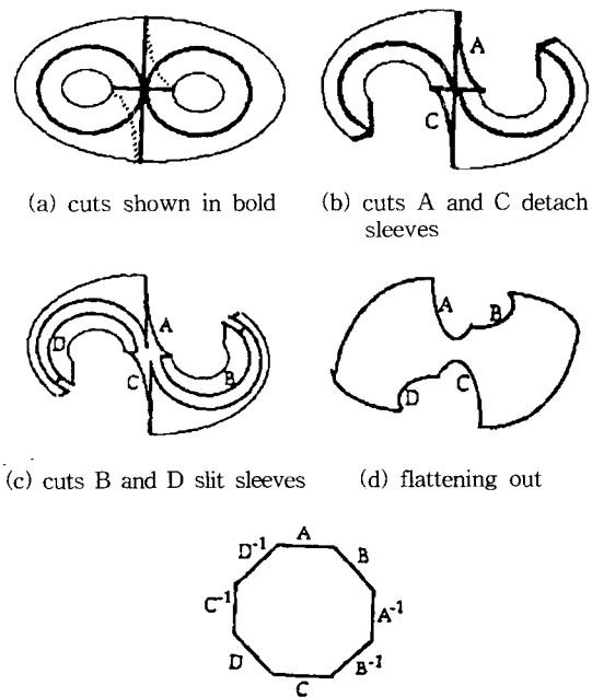
Fig. 1. Peeling a double torus
