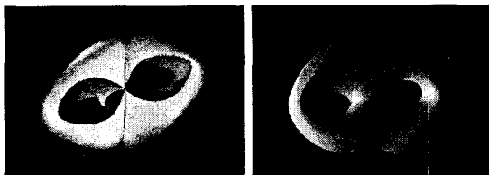
Fig. 3. multiperiodizing transformation
