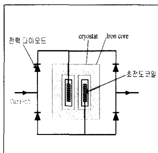
그림 4 초전도한류기
