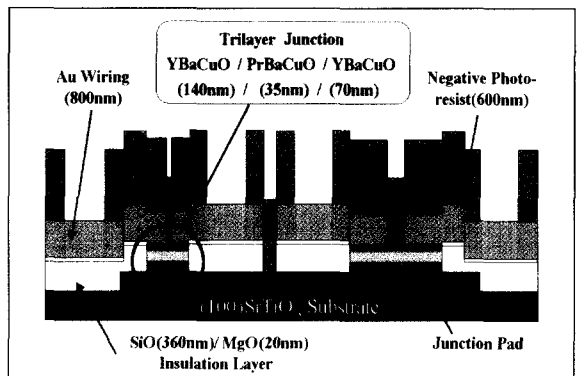
그림 6 초전도디지털소자
