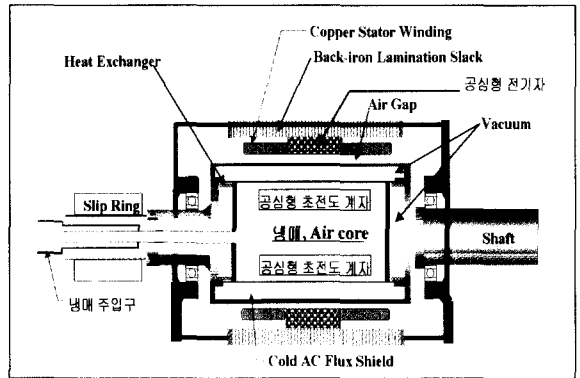
그림 5 초전도모터
