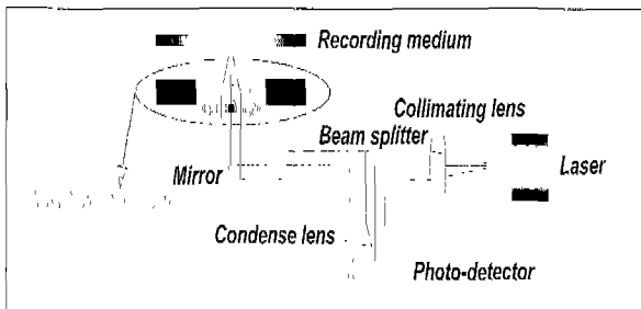
그림 7. 마이크로 렌즈의 위치제어를 통한 광기록 장치로의 응용 개념도. 마이크로 렌즈가 좌우로 움직이면 렌즈를 통과한 빛이 좌우로 위치를 변동하게 되어서 track-following이 가능하다.
