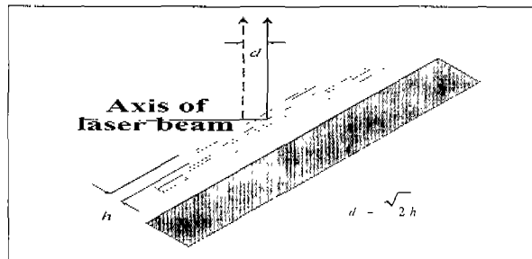
그림 8. 마이크로 미러를 이용하여 광기록 장치의 트랙 추종을 하는 Beam steering 원리
