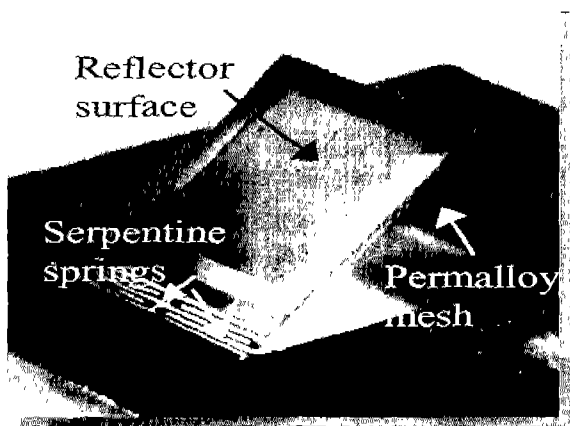
그림 10. 홀로그래프 정보저장 장치에 응용하는 4 mm 크기의 마이크로 미러. 자기력에 의해서 구동한다.
