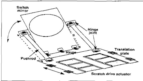
그림 15. SDA로 구동되는 마이크로 미러. 기판에 누워있다가 SDA가 닿기면 힌지 조인트 구조로 인해 마이크로 미러가 기판에 수직하게 서게 된다.
