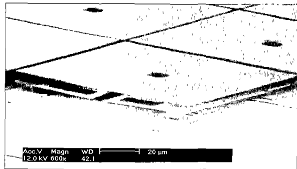
그림 17. 제작한 위상 변조용 알루미늄 마이크로 미러 어레이의 확대도. 크기는 100 μm / 100 μm 이다.
