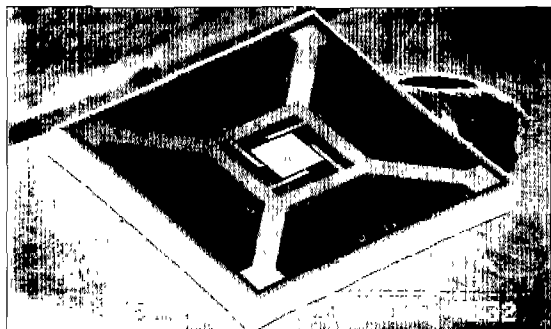
그림 9. 제작된 마이크로 미러와 액추에이터. 마이크로 미러의 한변의 크기는 500 \mu\text{m} 이다.
