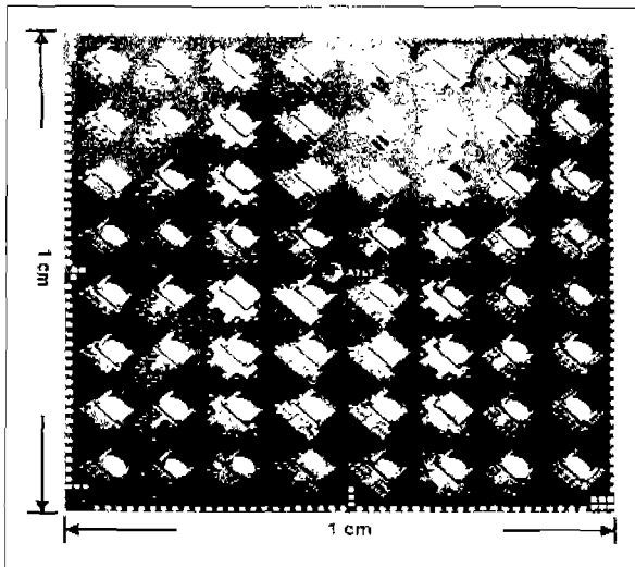
그림 16. 1 cm x 1 cm 의 크기 칩에 8 x 8 개 마이크로 미러가 제작된 예. 각 마이크로 미러의 구조는 그림 15와 같다.
