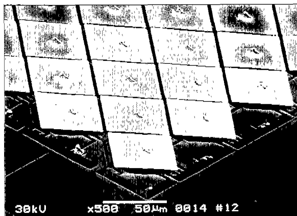
그림 13 알루미늄 표면 마이크로머시닝 기술로 제작한 마이크로 미러 어레이. 마이크로 미러의 크기는 50 \mu\text{m} 이다.
