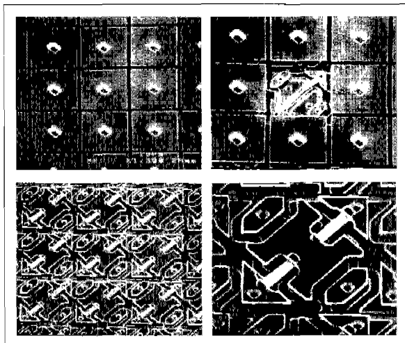
그림 12 알루미늄 마이크로머시닝으로 제작한 마이크로 미러 어레이
