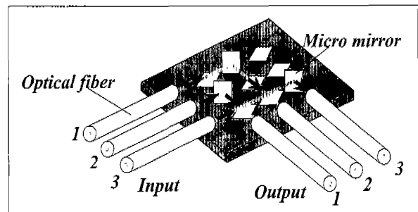
그림 14. 마이크로머시닝 기술로 제작하는 광 교환기의 개념도. 누워있던 마이크로 미러가 기판에 수직으로 서면 입력 광섬유로부터의 광을 반사하여 출력 광섬유로 내보낸다.
