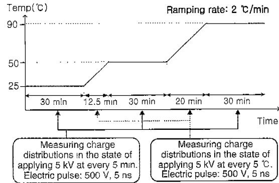
그림 1. 온도조절이 가능한 PEA system에서의 측정 과정 개략도.
