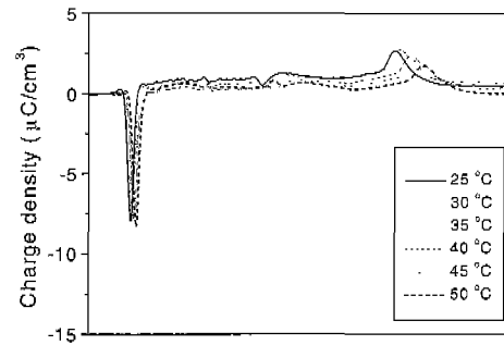
그림 5. 온도 변화에 따른 SXLPE/XLPE laminate의 전하 분포(5 kV 인가 중에 측정, 25 °C ~ 50 °C).
