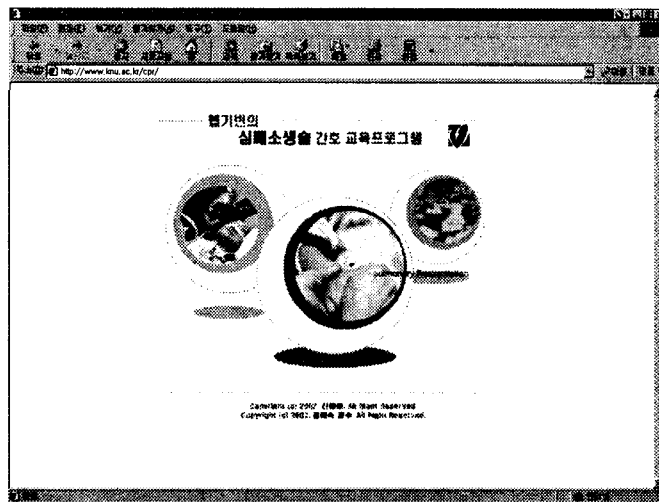
그림 1. 초기화면
