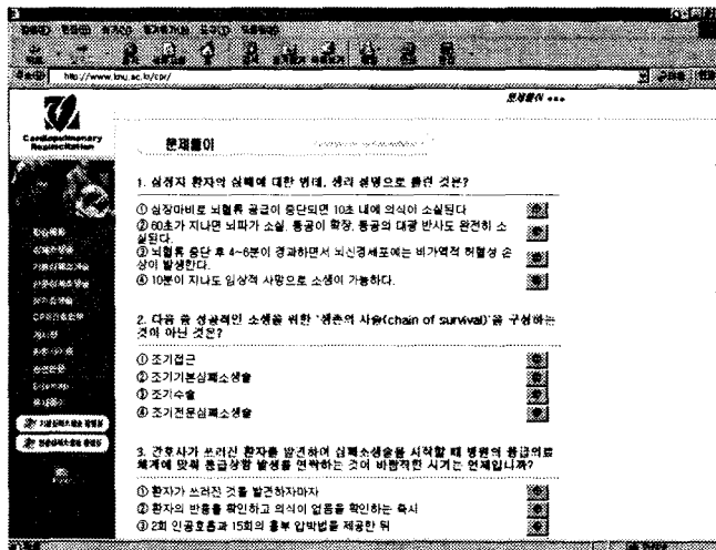
그림 5. 문제풀이 화면
