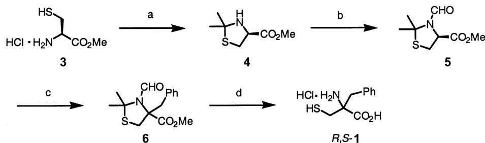
Scheme 1. (a) Et 3 N, Acetone, reflux, 24 h, 97%; (b) acetic anhydride, sodium formate, formic acid, rt, 10 h, 75%; (c) LDA, C 6 H 5 CH 2 Br, THF, -90 °C, 30%; (d) 6 N HCl, reflux, 48 h, 90%.
