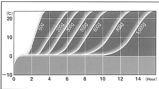
〈캐치쿨 보냉성능〉
