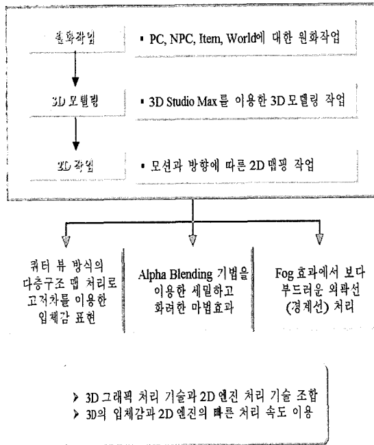
그림 10. 그래픽처리
