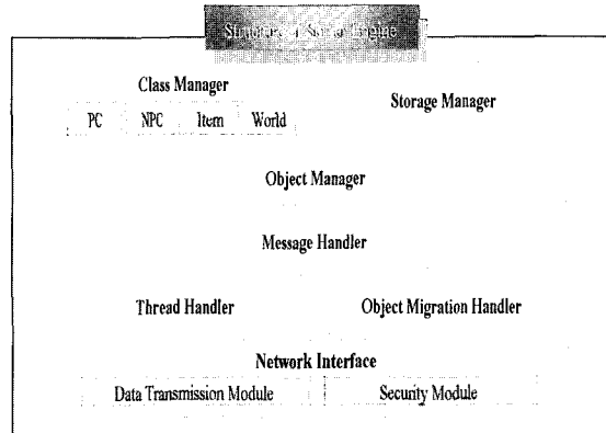
그림 2. 서버엔진 구조
