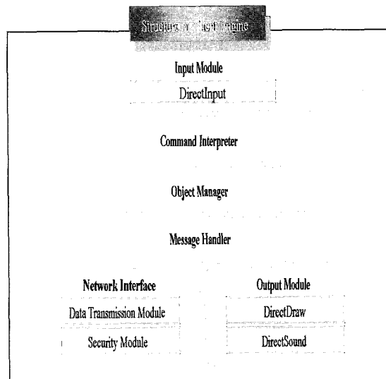
그림 8. 클라이언트엔진 구조
