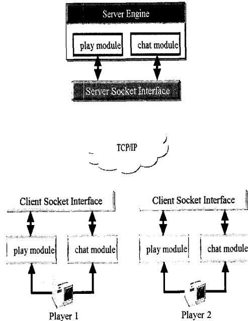
그림 11. Client-Server 통신처리
