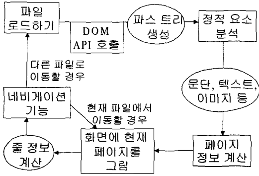
(그림 2) 시스템 구조도
