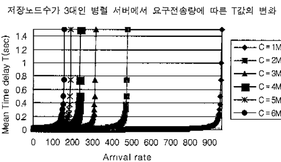
(그림 9) 저장노드수가 3대인 병렬 서버에서 요구전송량에 따른 T값의 변화
