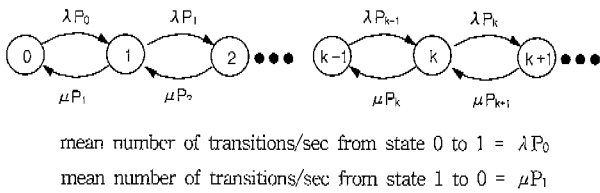
(그림 7) M/M/1 큐잉 모델의 상태 천이도
