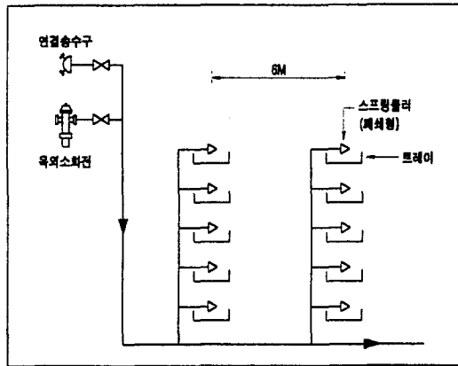
그림 2. 스프링클러+연결살수설비 혼합방식.
