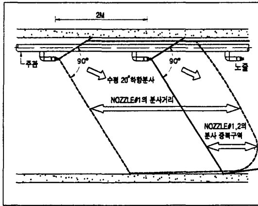
그림 5. 워터미스트 노즐의 분사시 확산범위.
