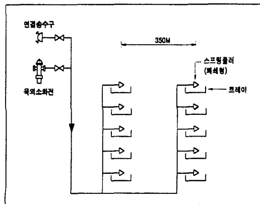
그림 3. 연소방지형 소화설비 방식.
