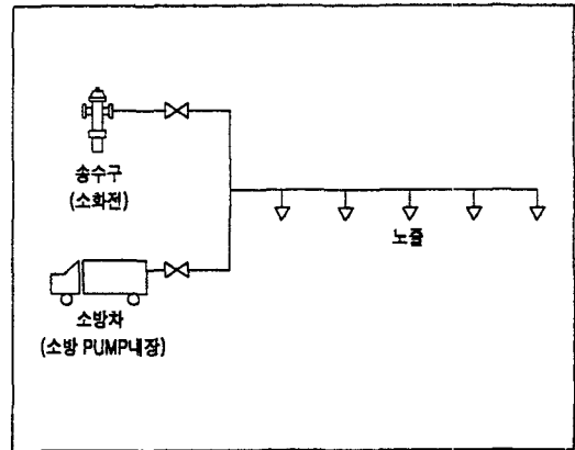
그림 1. 공동구의 소화설비 기본방향.
