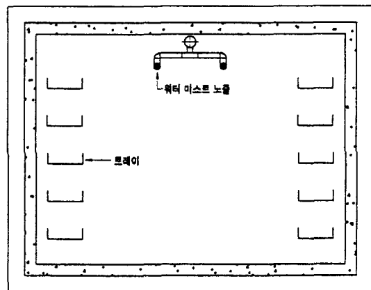
그림 4. 워터 미스트 설치 상세도.
