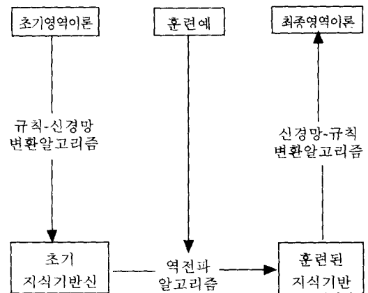
그림 1. 지식기반신경망에서의 처리절차
