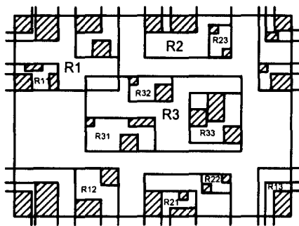
그림 1. CR-트리의 검색공간
