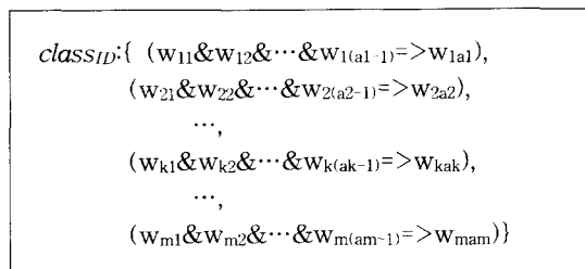
그림 4. 연관 단어 지식 베이스의 구조
