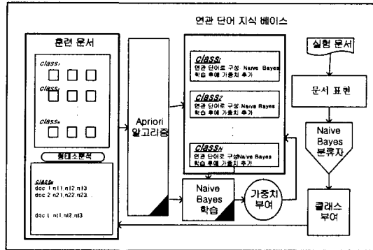
그림 5. 연관 단어 지식 베이스를 기반으로 하는 가중치가 부여된 베이지안 분류자의 구성도
