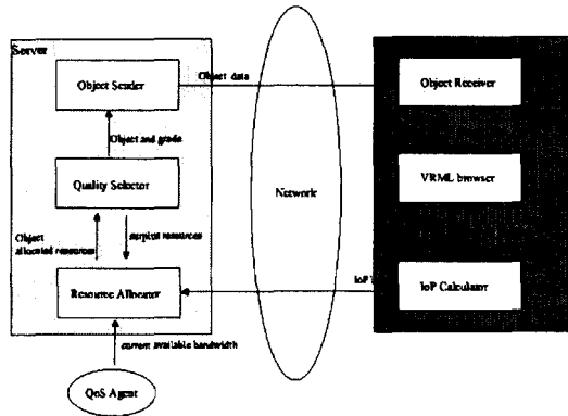
그림 4. 제안된 NVR 시스템의 구조
