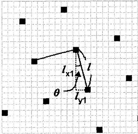
그림 5. 해프토닝시 파라미터에 따른 해프톤 셀 중심의 분포
