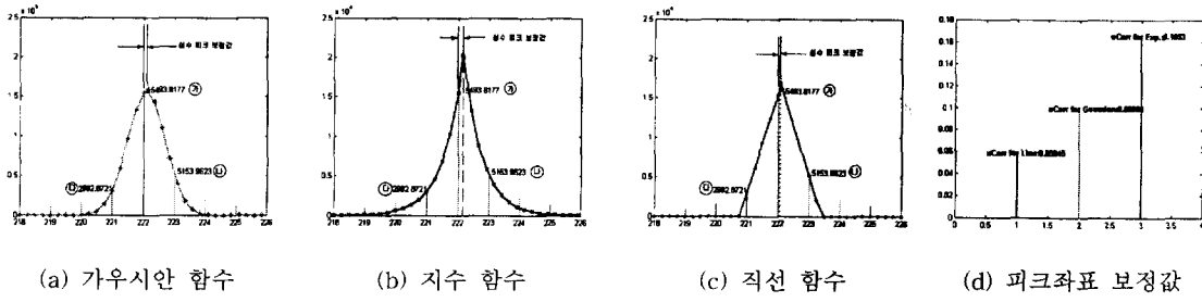
그림 11. 피크 모델링 방법 및 피크좌표 보정값
