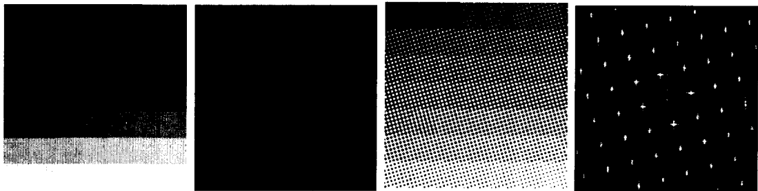
(a) 연속계조영상 (b) 연속계조영상의 푸리에 특성 (c) 해프톤 영상 (d) 해프톤 영상의 푸리에 특성
