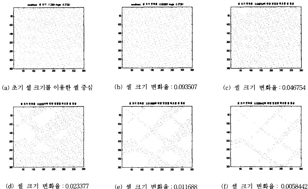
그림 13. 셀 크기 변화율에 따라 변경된 셀 중심
