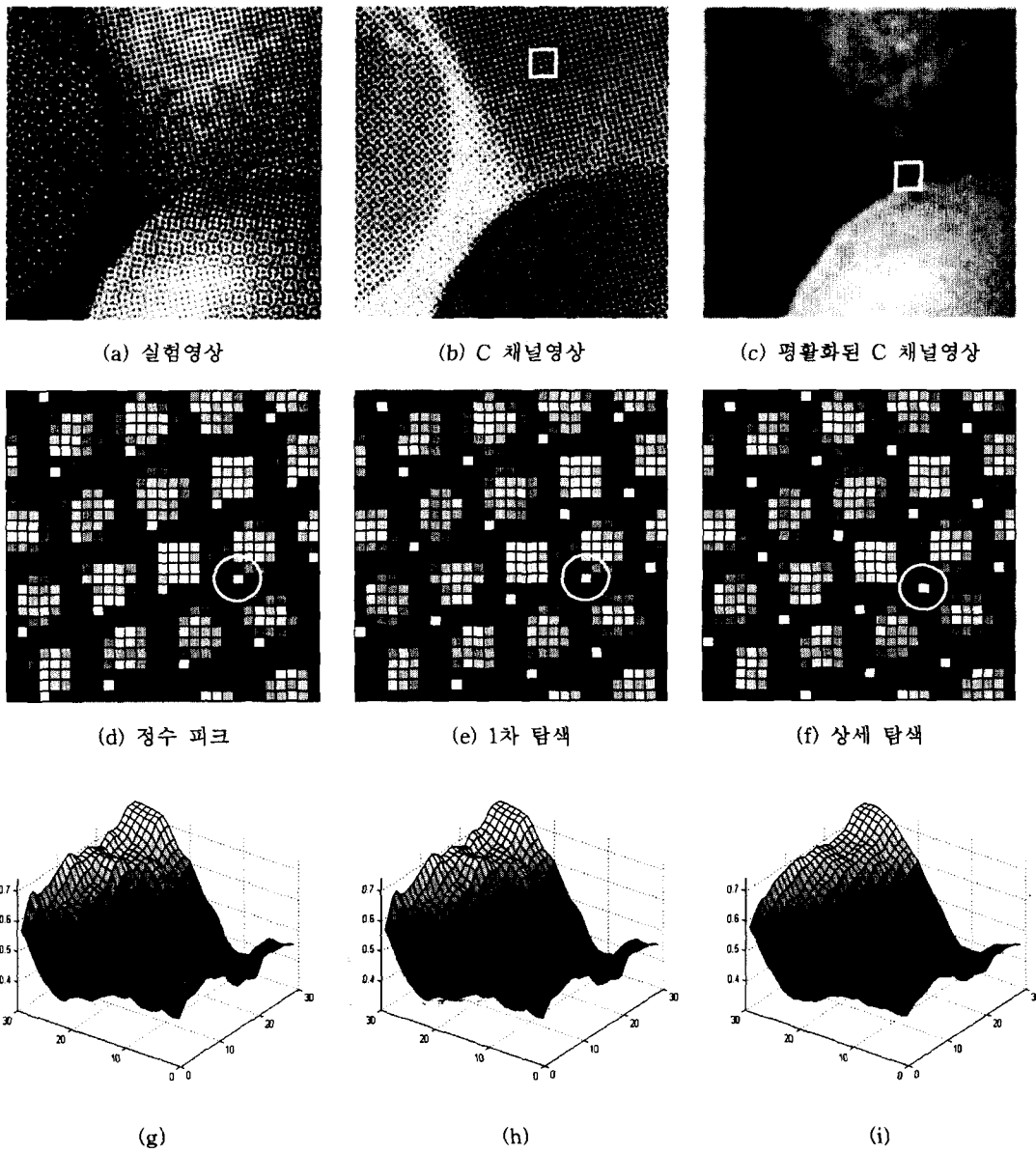
그림 16. 셀 크기가 큰 경우의 헤프톤 셀 중심 추출 결과 비교
